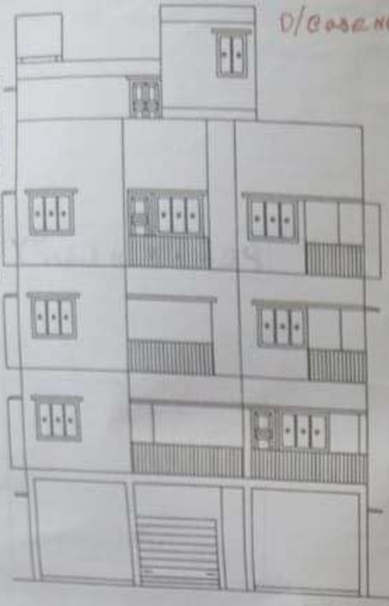
FRONT ELEVATION SCALE: 1/50
